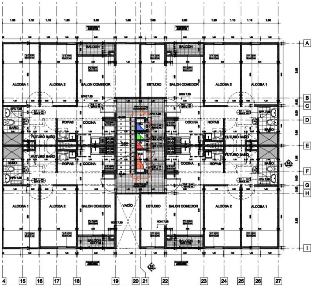
ARQUITECTÓNICO- PISO 4- TORRE 1
