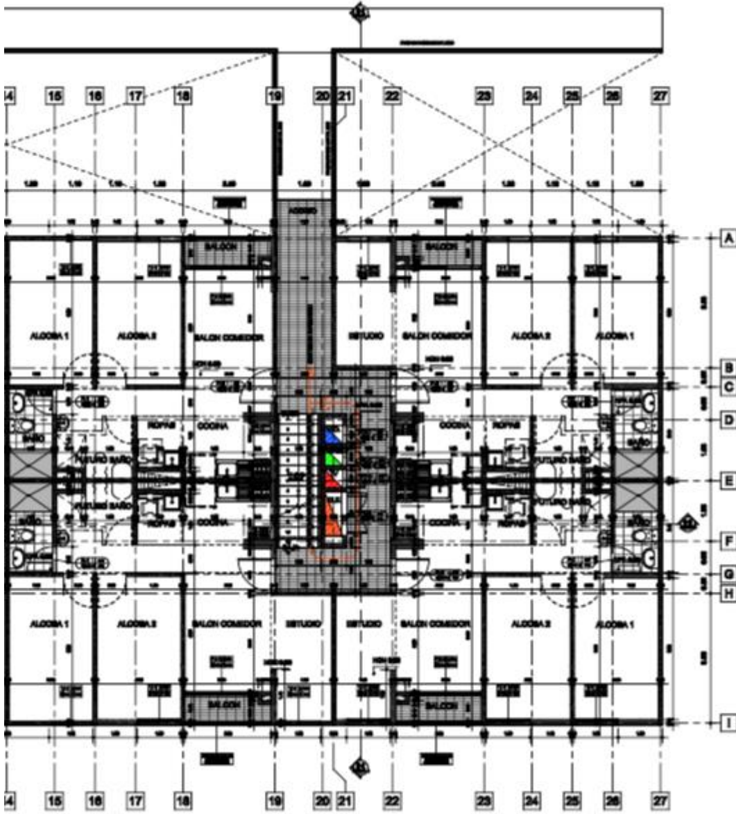
ARQUITECTÓNICO- PISO 1- TORRE 1
