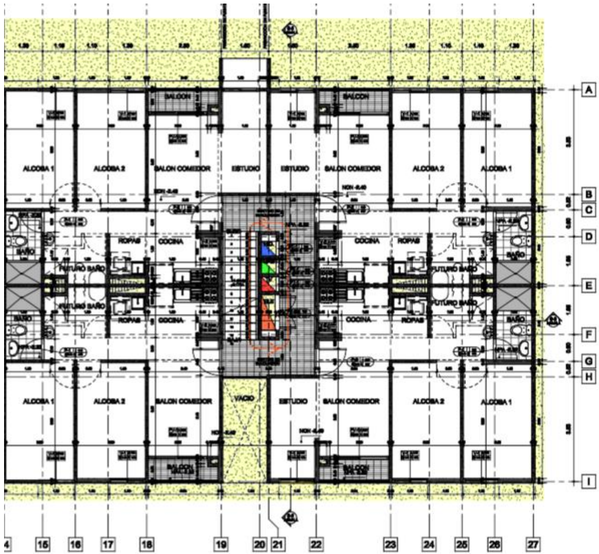
ARQUITECTÓNICO- PISO 99- TORRE 1
