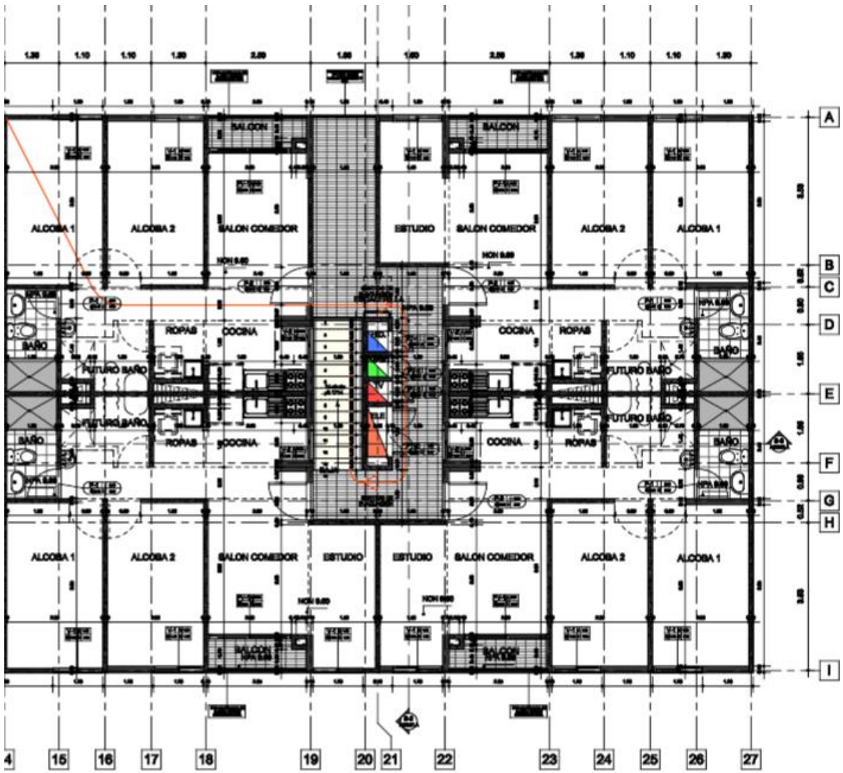
ARQUITECTÓNICO- PISO 5- TORRE 1
