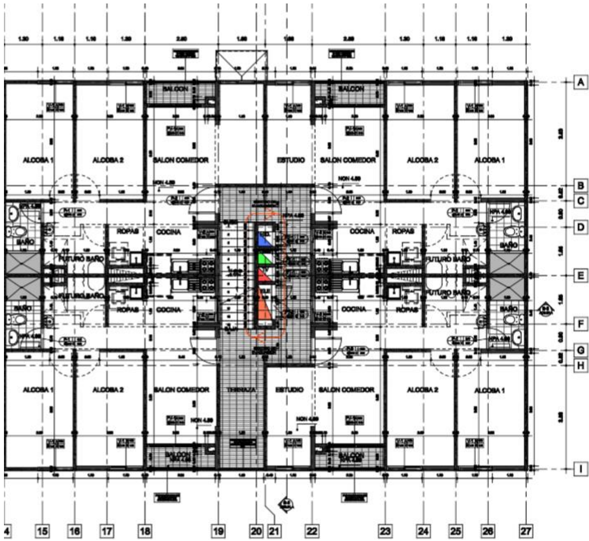
ARQUITECTÓNICO- PISO 3- TORRE 1
