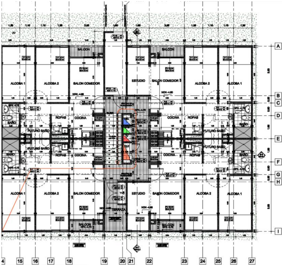
ARQUITECTÓNICO- PISO 98- TORRE 1
