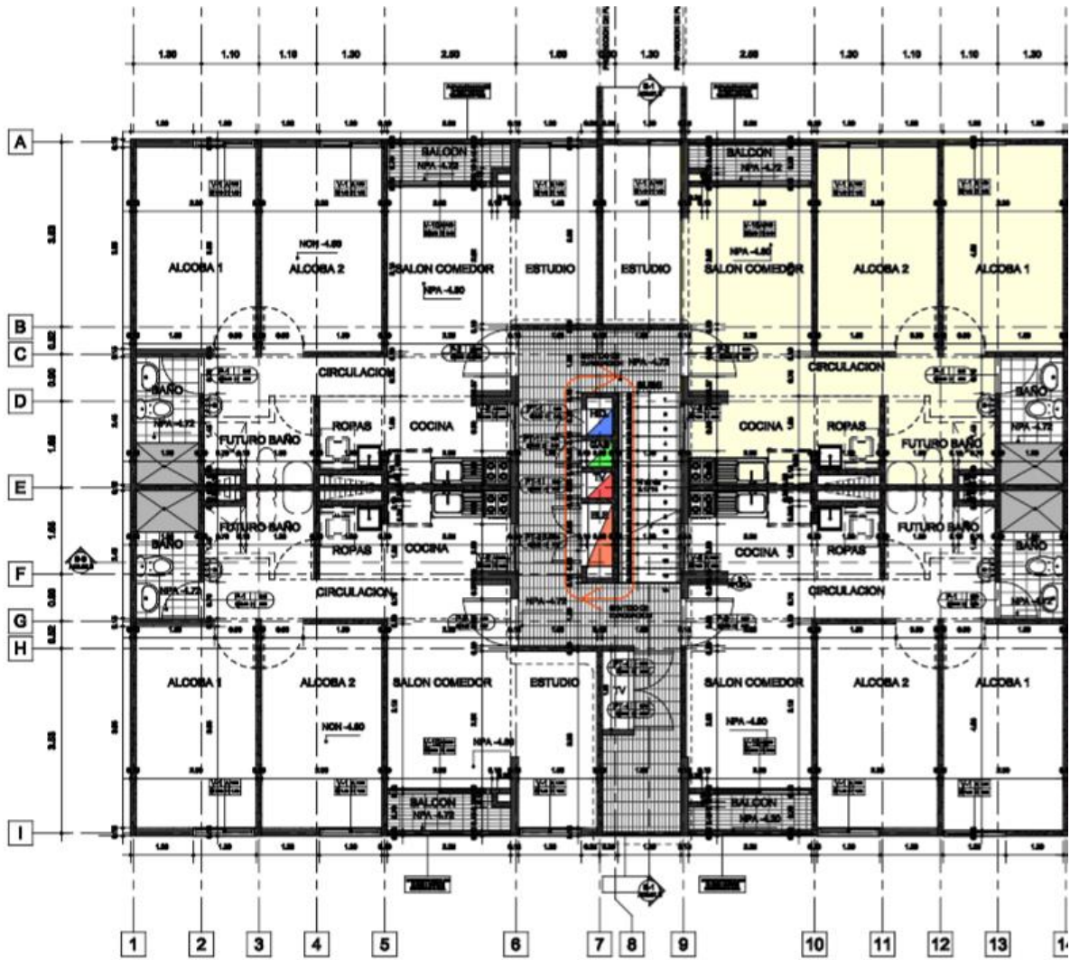
ARQUITECTÓNICO- PISO 98- TORRE 4
