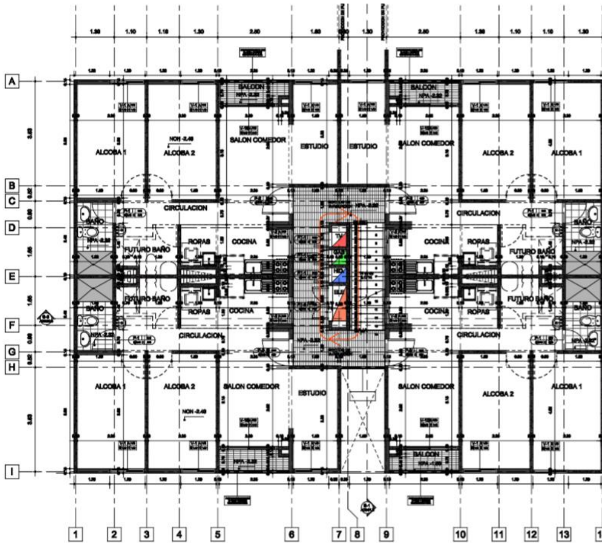
ARQUITECTÓNICO- PISO 99- TORRE 4
