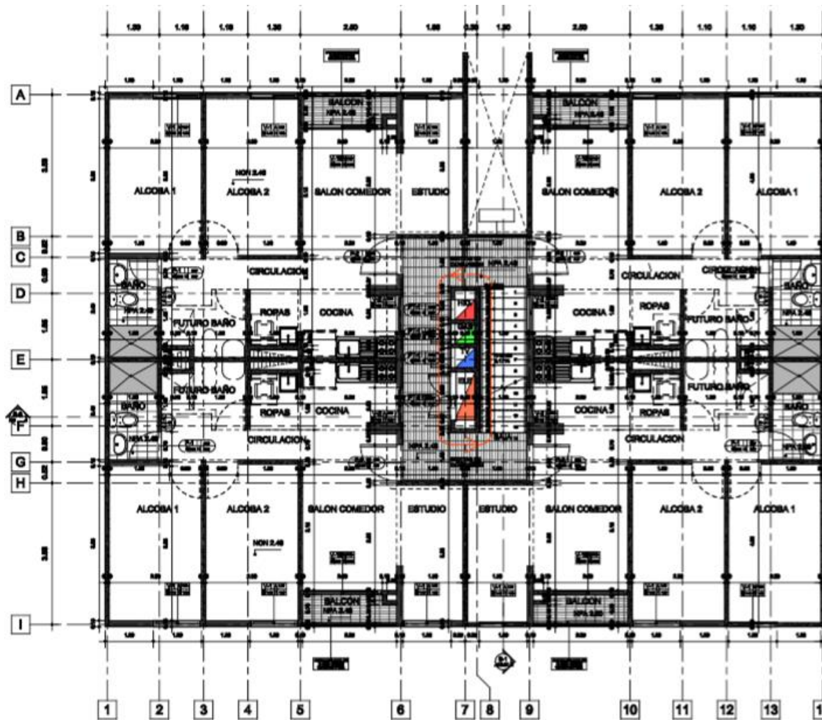
ARQUITECTÓNICO- PISO 2- TORRE 4
