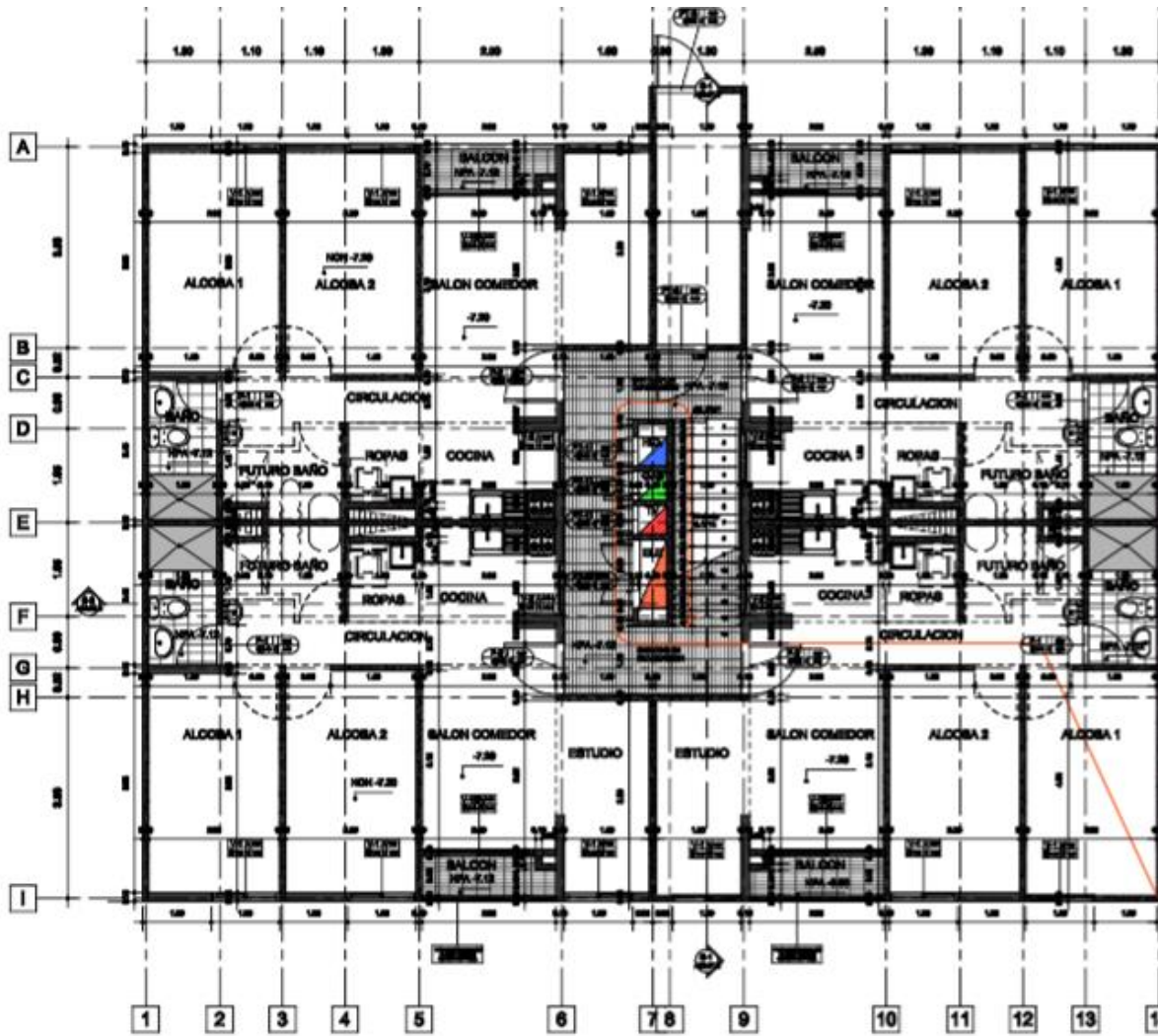
ARQUITECTÓNICO- PISO 97- TORRE 4
