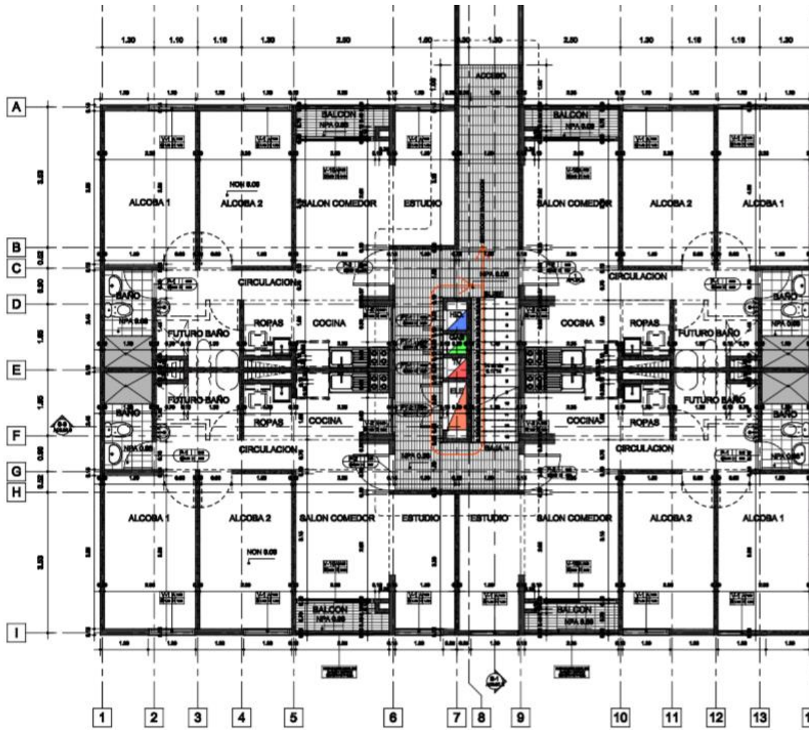
ARQUITECTÓNICO- PISO 1- TORRE 4
