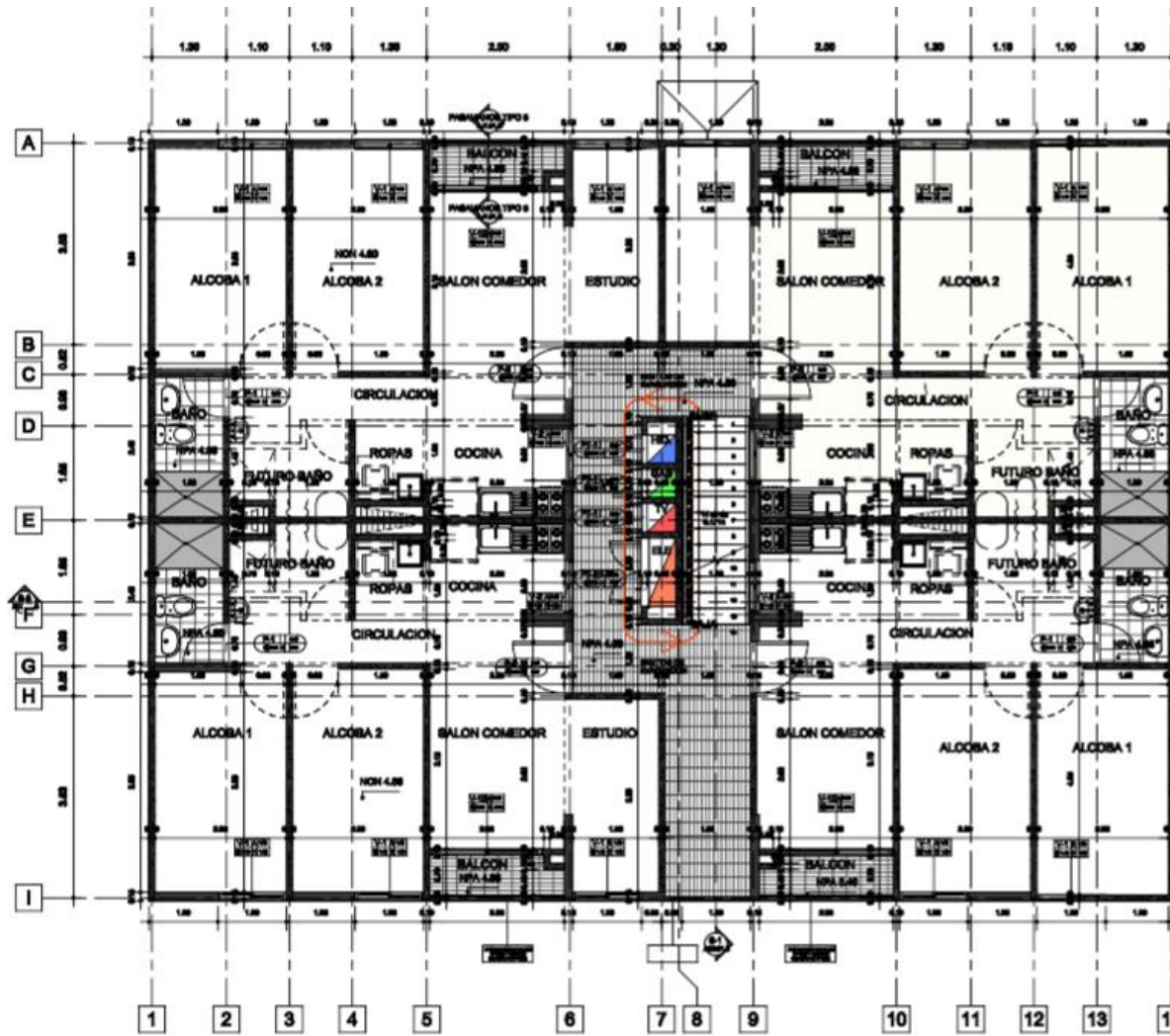
ARQUITECTÓNICO- PISO 3- TORRE 4
