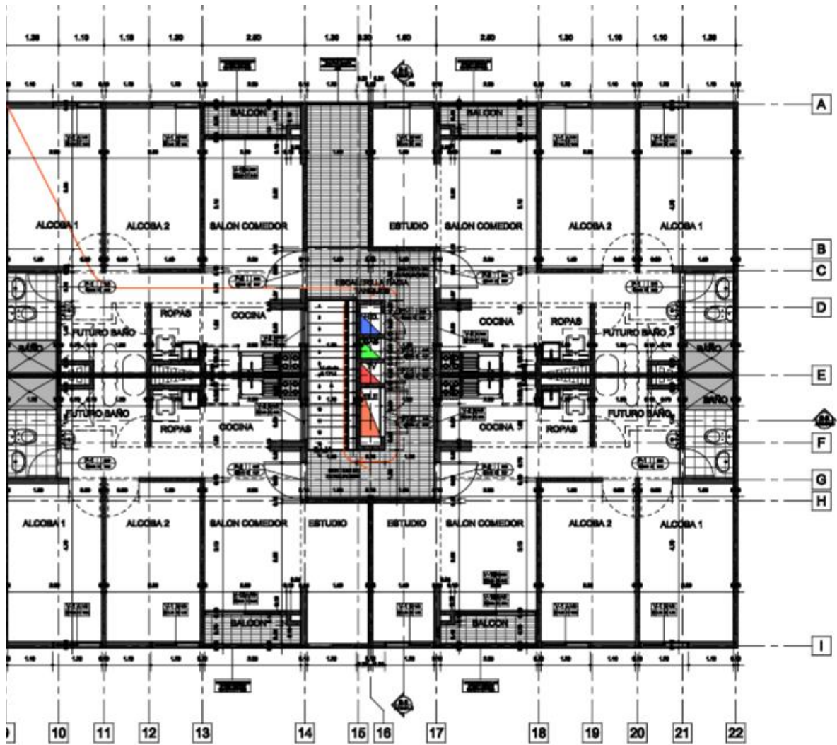
ARQUITECTÓNICO- PISO 5- TORRE 5
