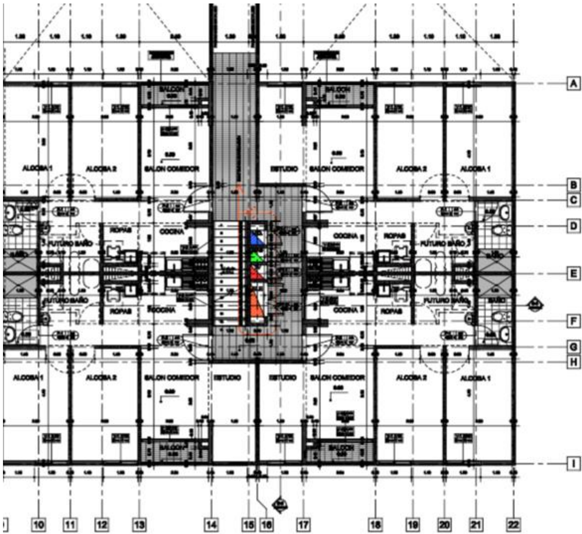
ARQUITECTÓNICO- PISO 1- TORRE 5
