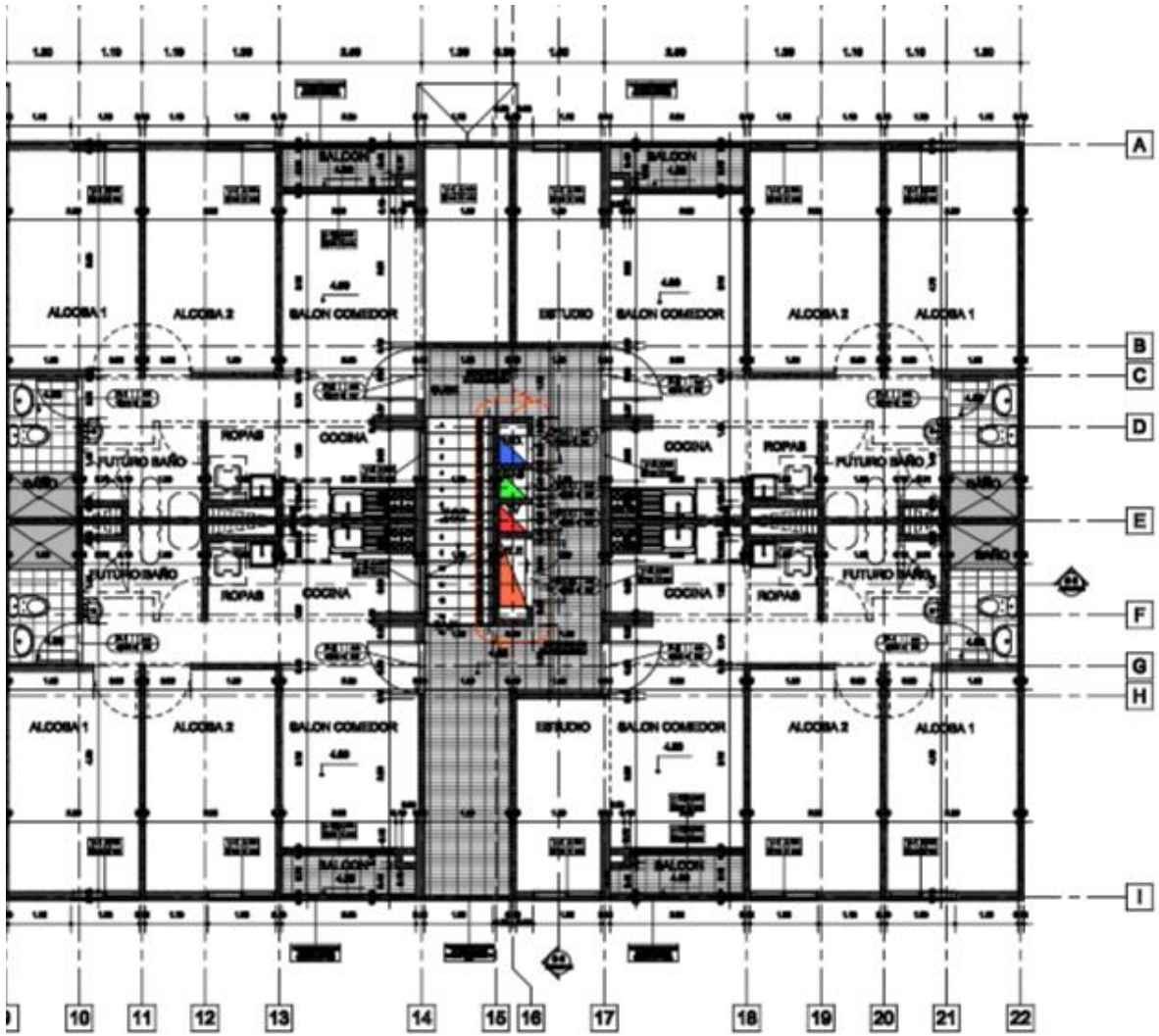
ARQUITECTÓNICO- PISO 3- TORRE 5
