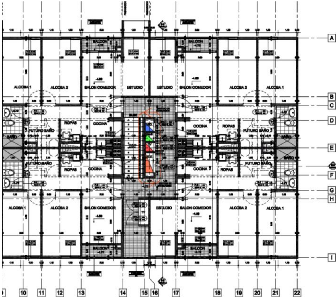
ARQUITECTÓNICO- PISO 98- TORRE 5
