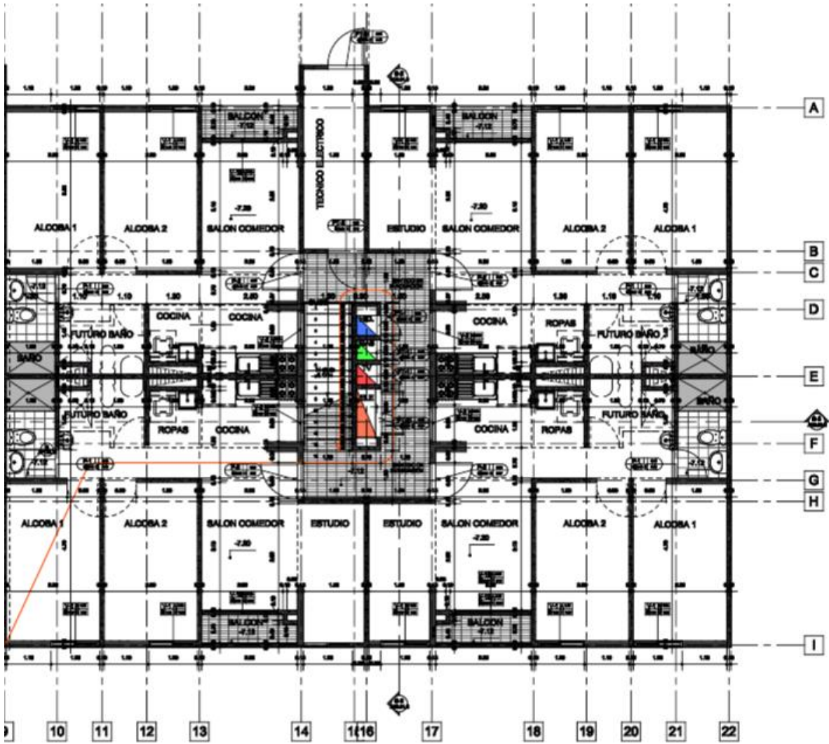
ARQUITECTÓNICO- PISO 97- TORRE 5
