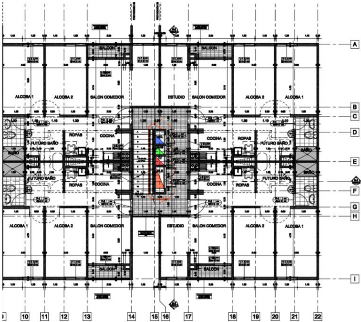
ARQUITECTÓNICO- PISO 99- TORRE 5
