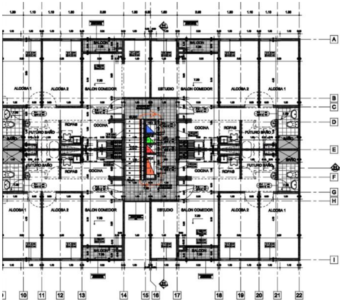
ARQUITECTÓNICO- PISO 4- TORRE 5
