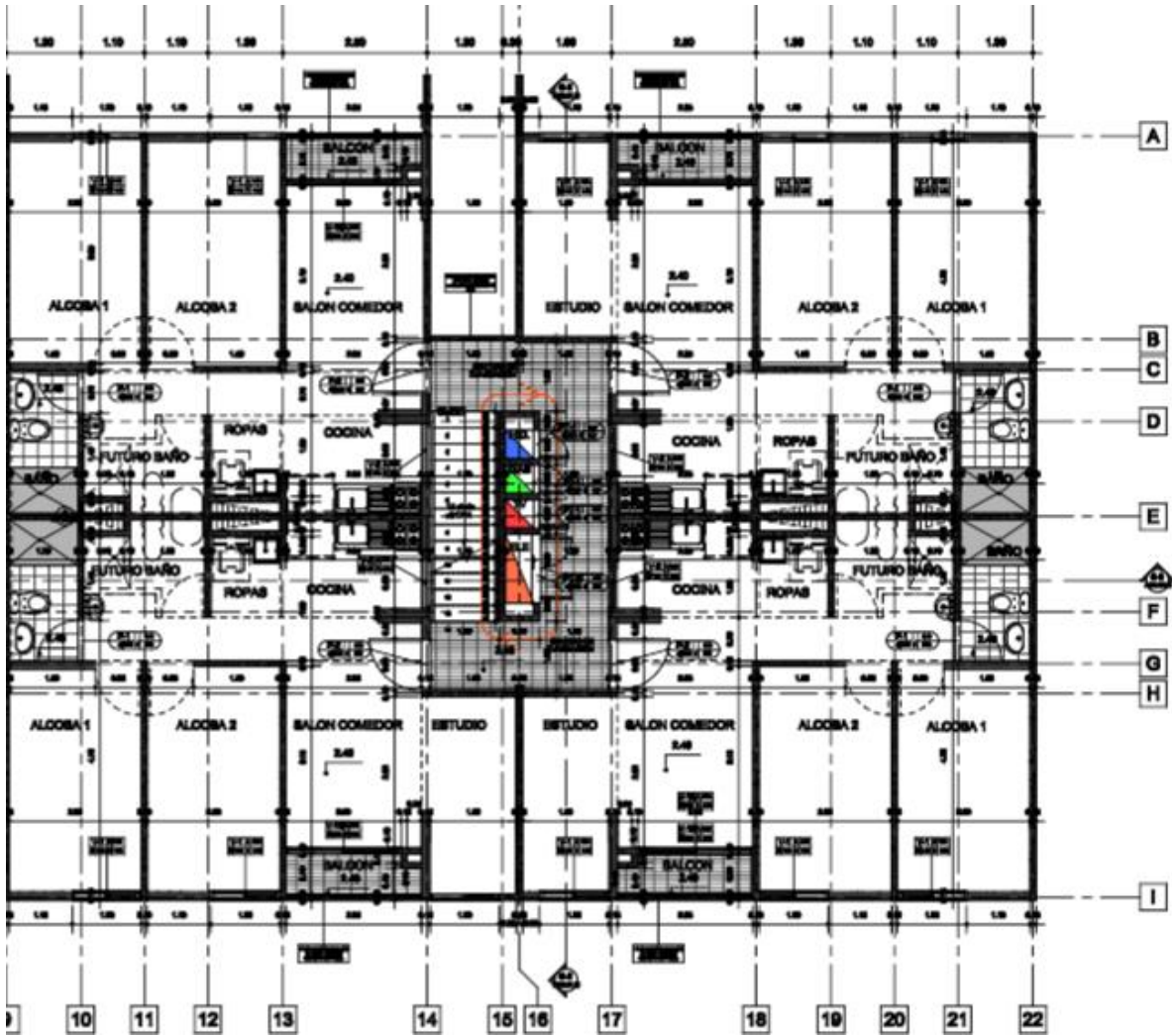
ARQUITECTÓNICO- PISO 2- TORRE 5
