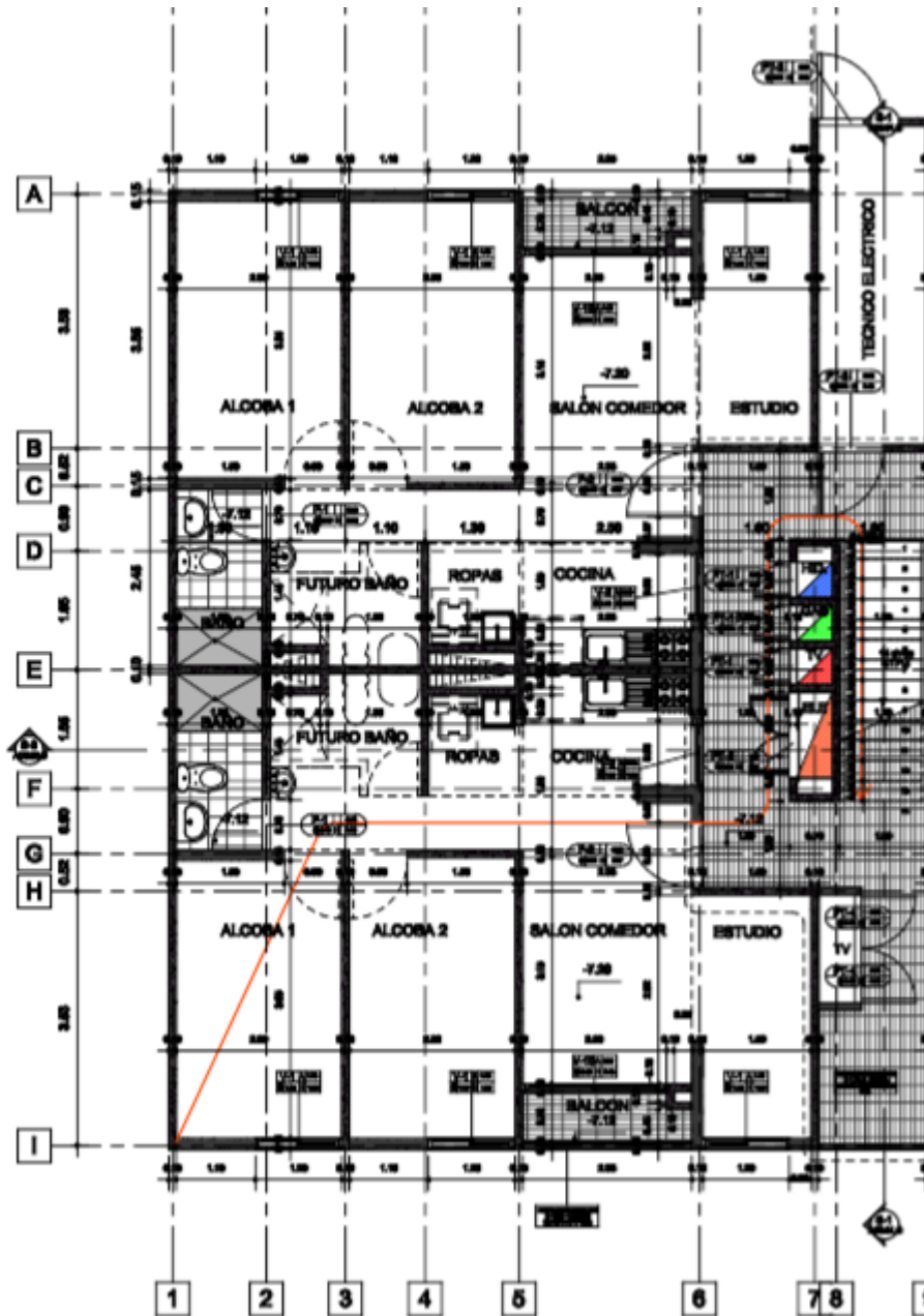
ARQUITECTÓNICO- PISO 97- TORRE 6
