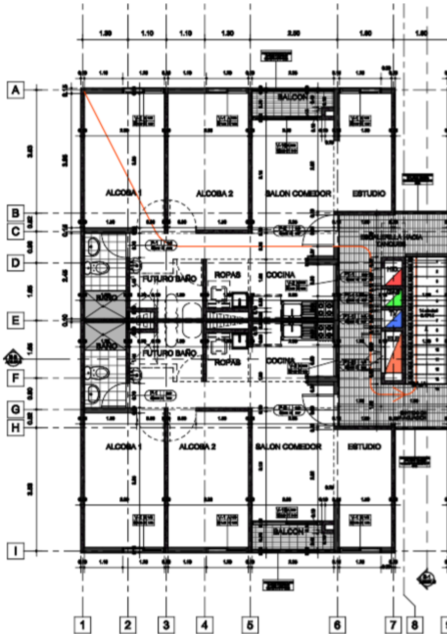
ARQUITECTÓNICO- PISO 5- TORRE 6
