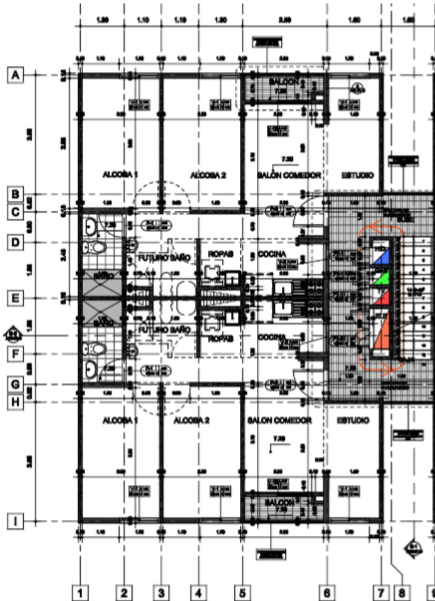
ARQUITECTÓNICO- PISO 4- TORRE 6
