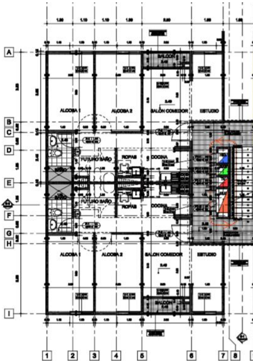
ARQUITECTÓNICO- PISO 2- TORRE 6
