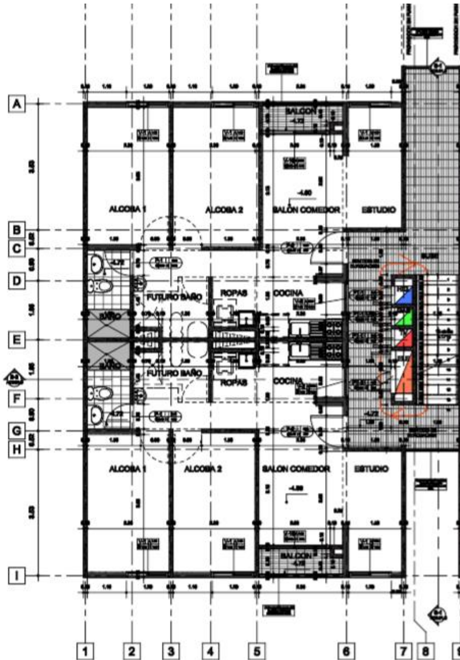
ARQUITECTÓNICO- PISO 98- TORRE 6
