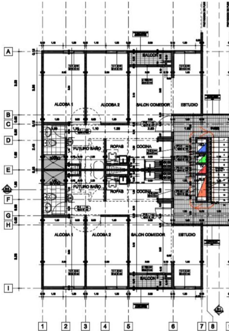
ARQUITECTÓNICO- PISO 99- TORRE 6
