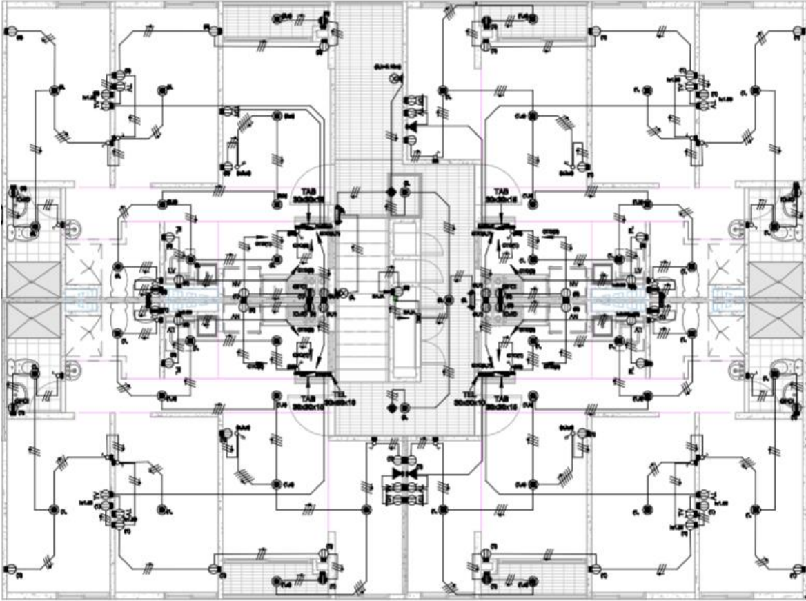
ELECTRICO- PISO 5- TORRE 5
