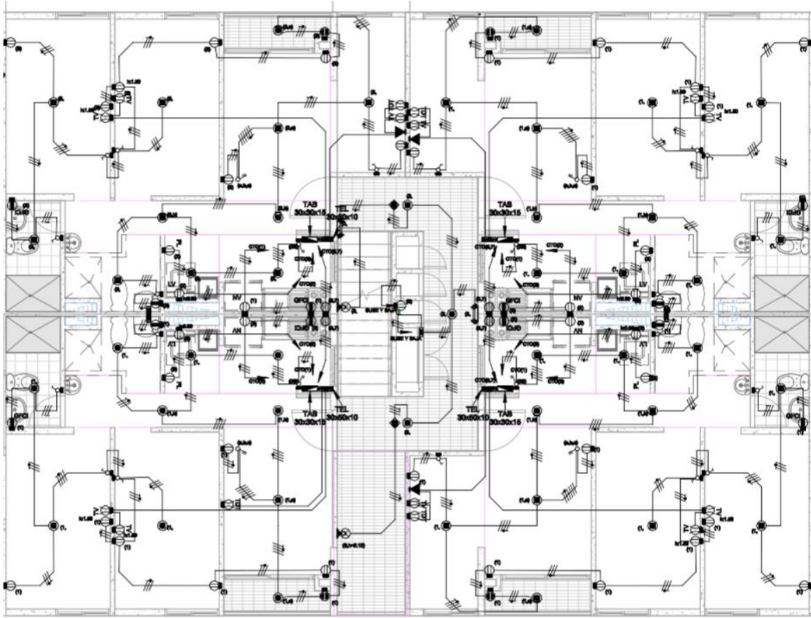
ELECTRICO- PISO 3- TORRE 5
