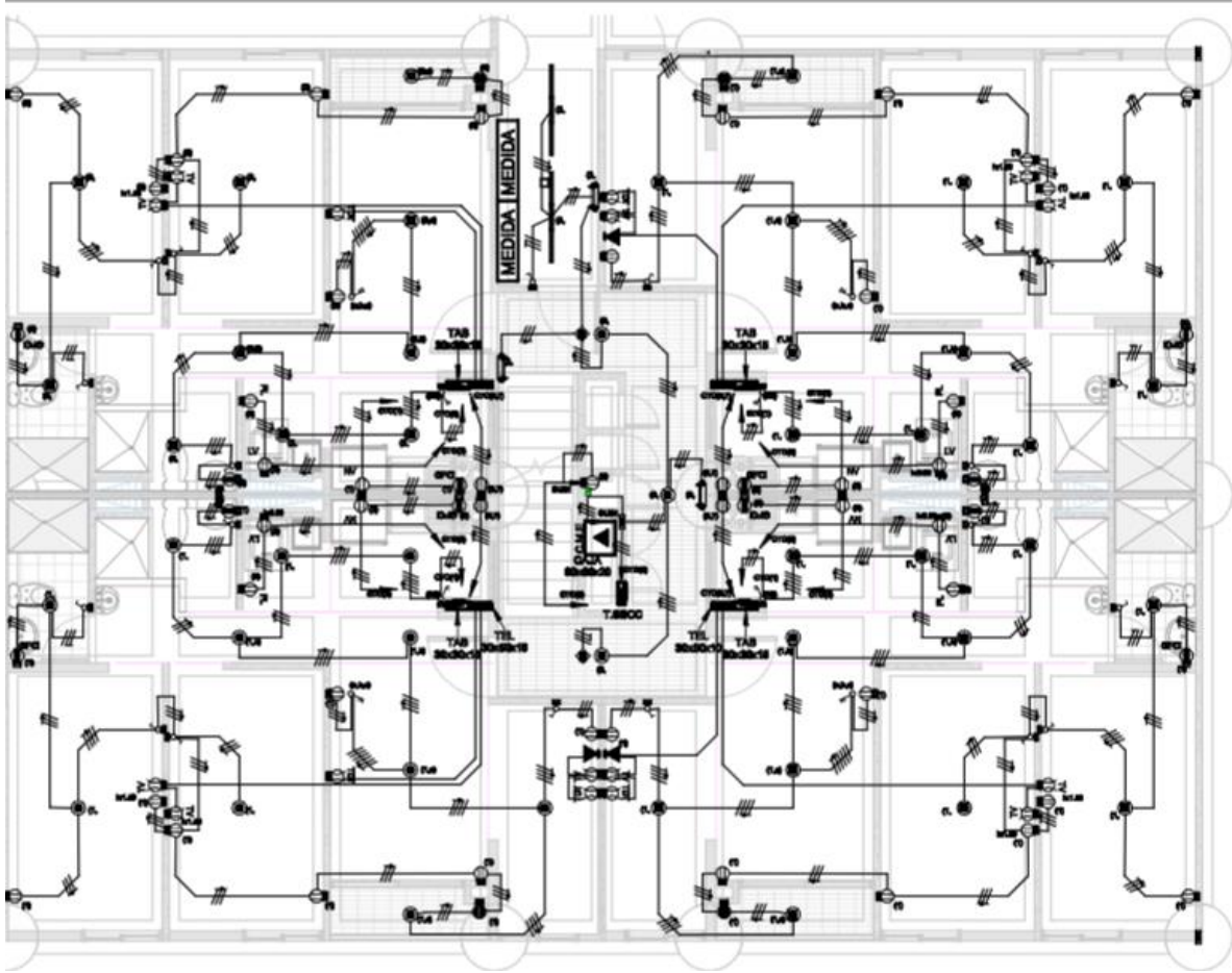
ELECTRICO- PISO 97- TORRE 5
