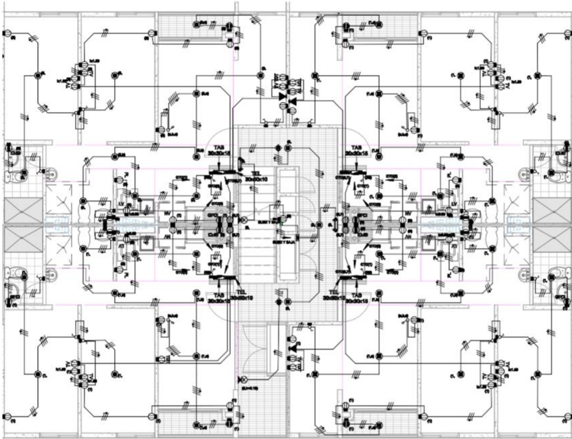
ELECTRICO- PISO 98- TORRE 5
