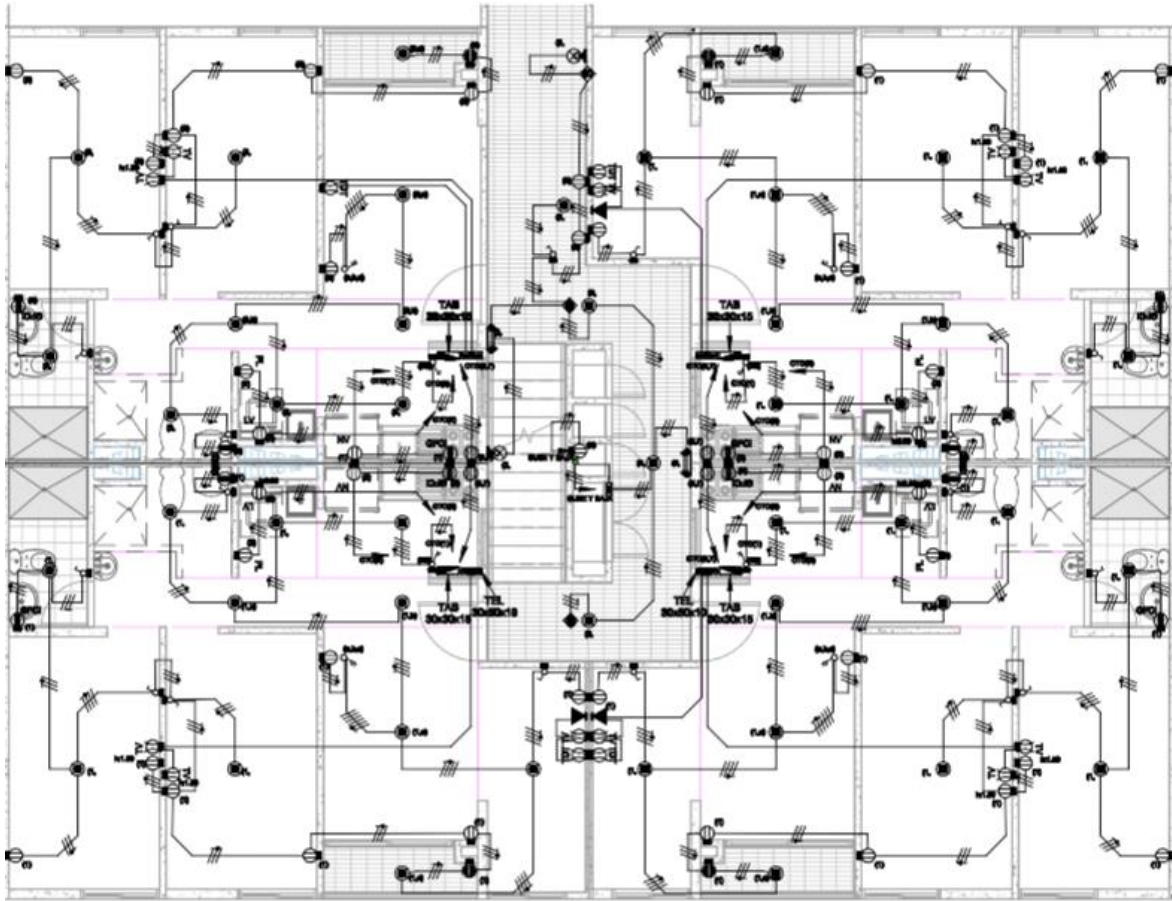
ELECTRICO- PISO 1- TORRE 5
