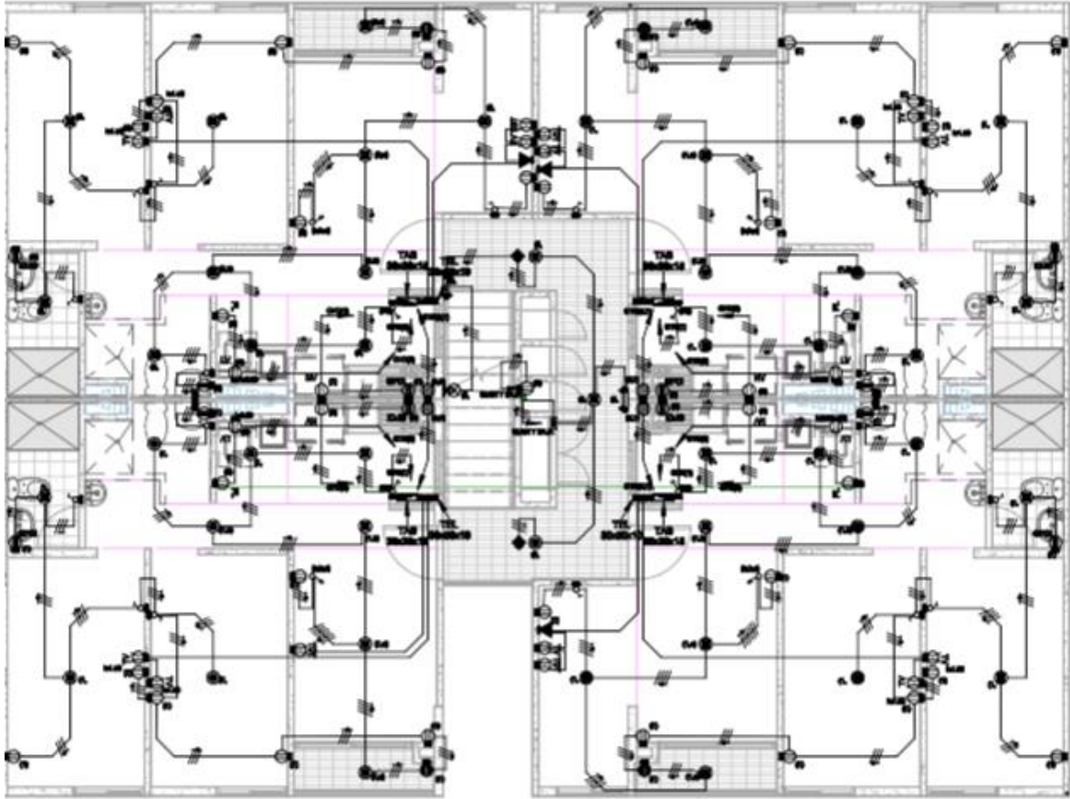
ELECTRICO- PISO 4- TORRE 5
