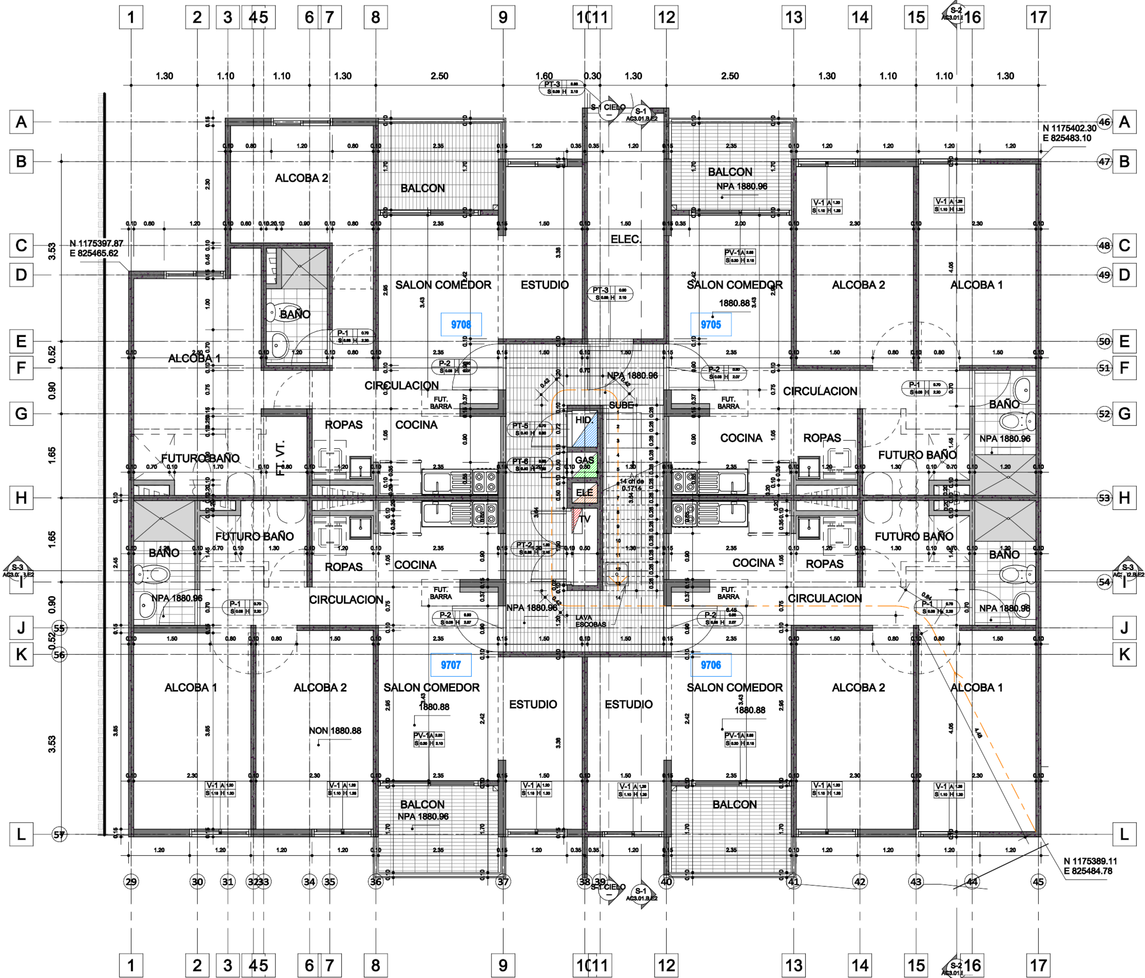
PLANTA PISO 97 1 : 50
