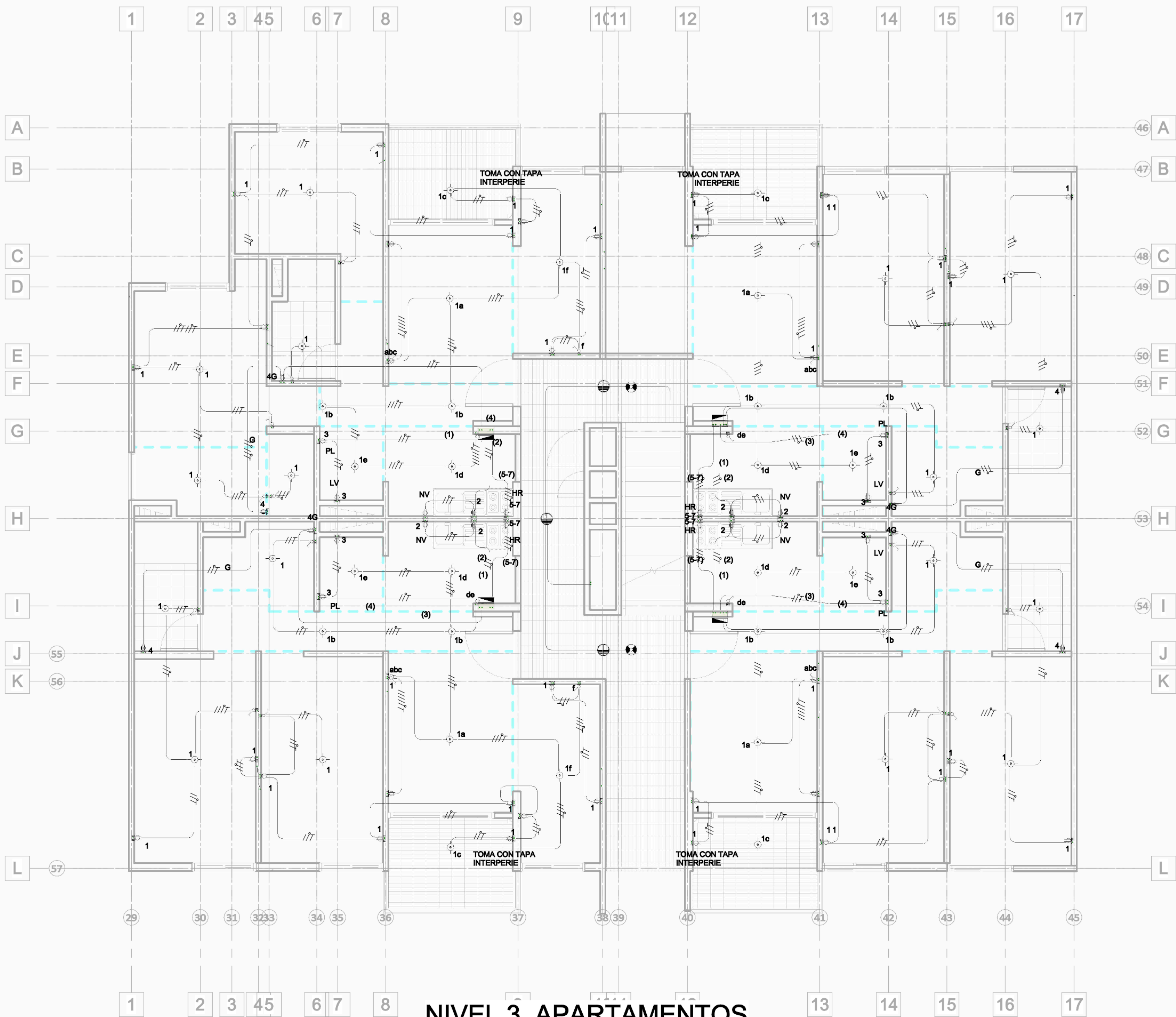
NIVEL 3 APARTAMENTOS ILUMINACIÓN Y TOMAS ESCALA 1:50
