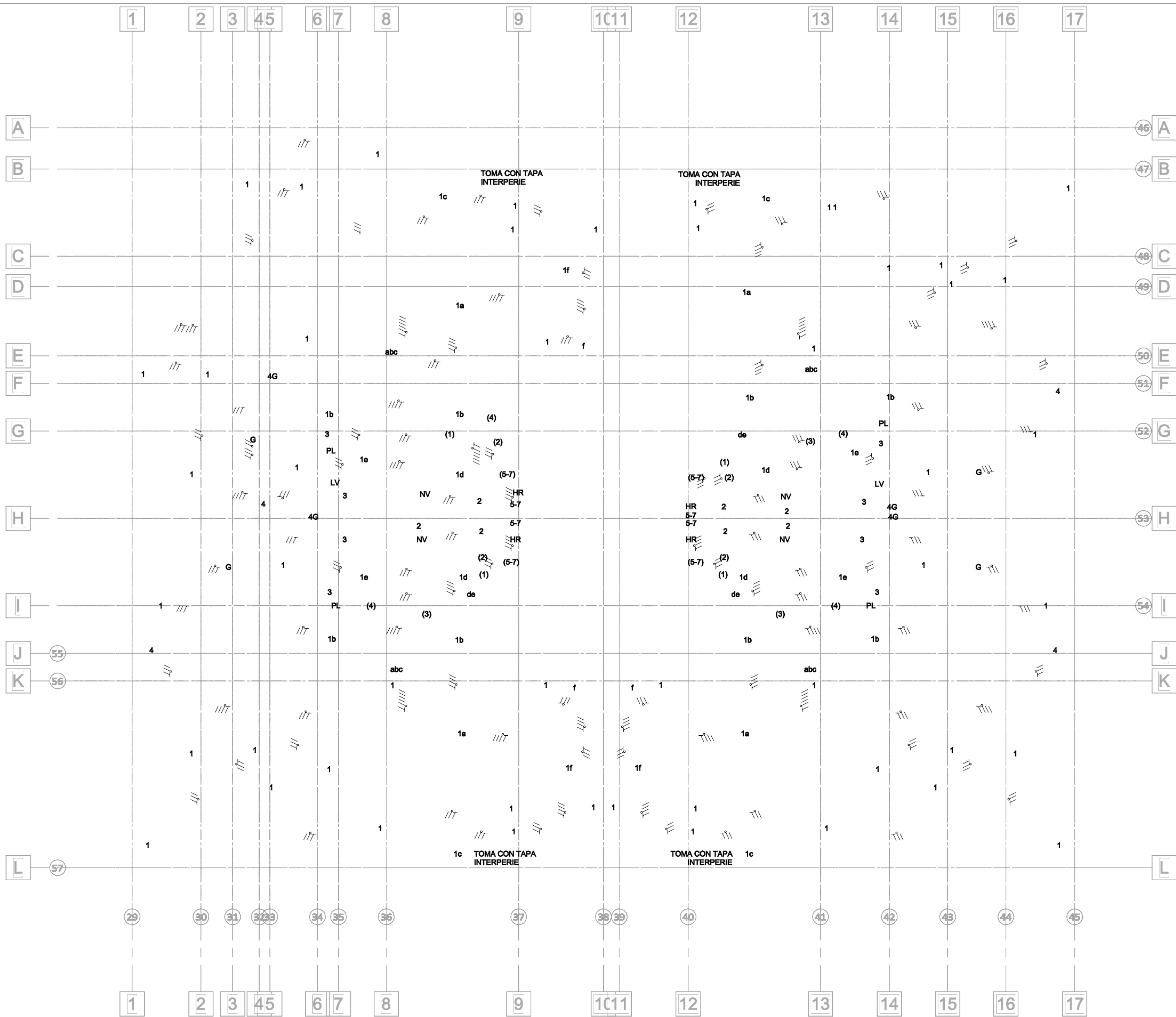
NIVEL 5 APARTAMENTOS ILUMINACIÓN Y TOMAS ESCALA 1:50
