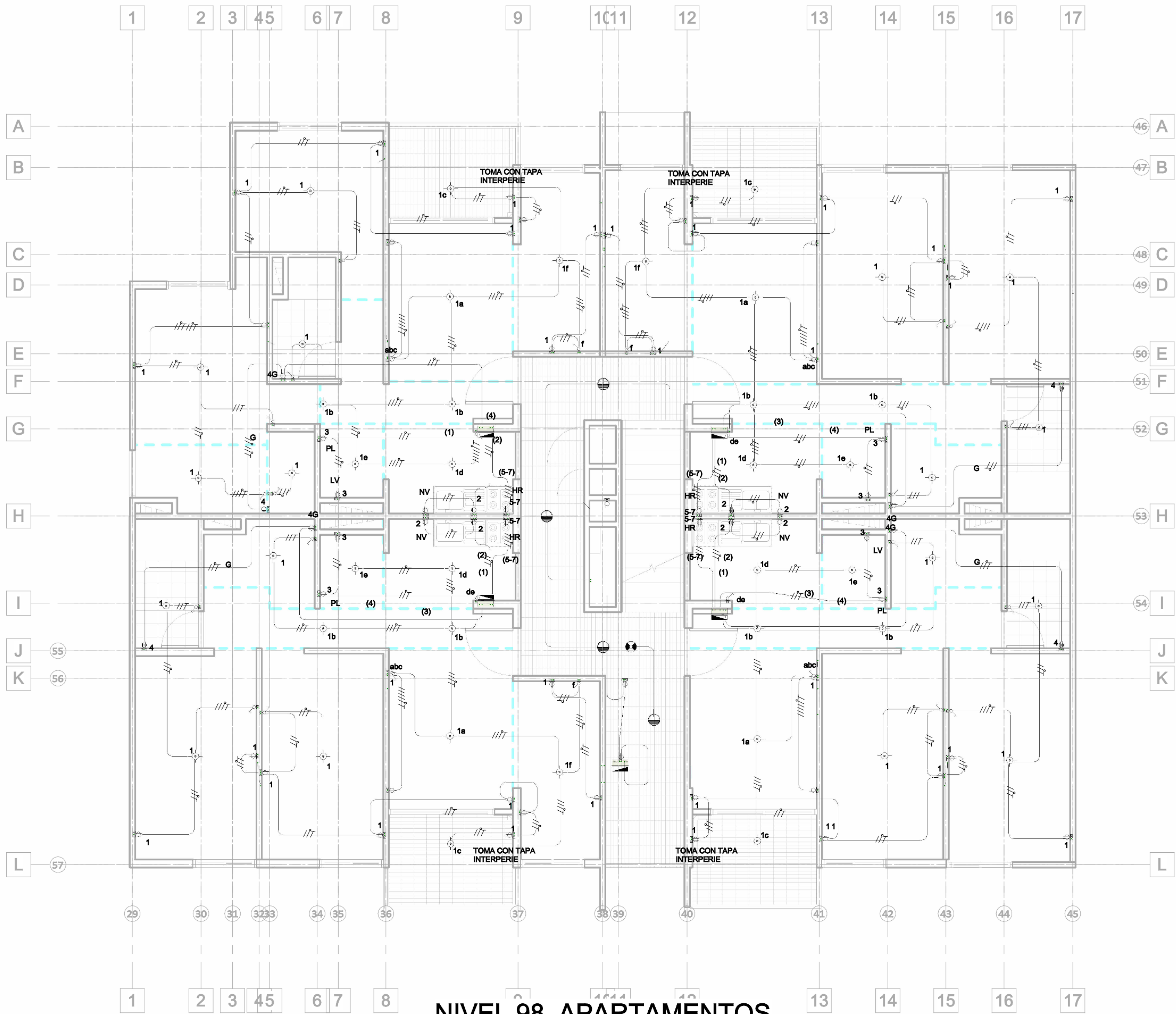
NIVEL 98 APARTAMENTOS ILUMINACIÓN Y TOMAS ESCALA 1:50
